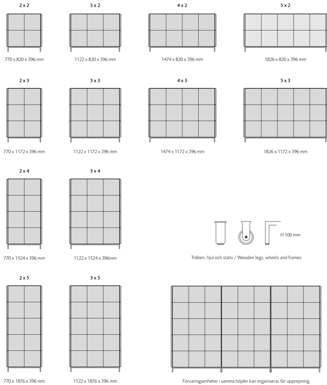
Förvaringsenheter i samma höjder kan organiseras för upprepning / Storage units with same heights can be performed for repetition
