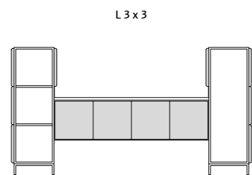
1826 x 1172 x 396 mm Bordshöjd / Table height 710 mm
