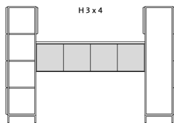
1826 x 1524 x 396 mm Bordshöjd / Table height 1040 mm
