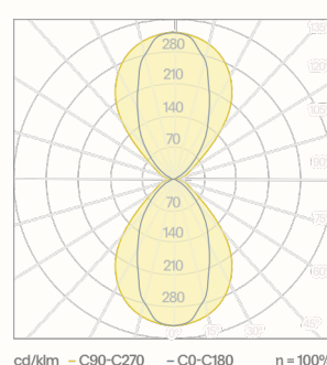
Polarintensitätsdiagramm
