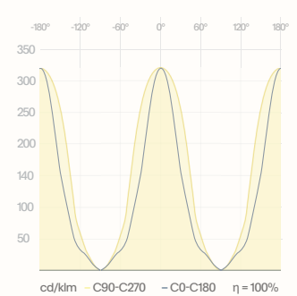
Lichtverteilung
