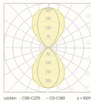
Polarintensitätsdiagramm
